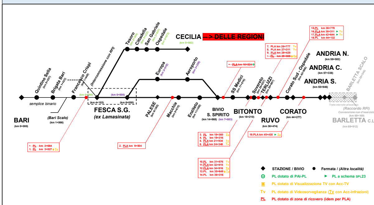
FIGURA 4: PASSAGGI A LIVELLO
