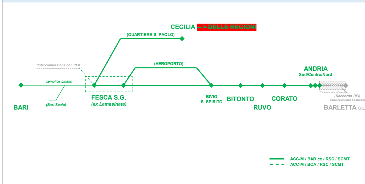
FIGURA 10: SISTEMI TECNOLOGICI DI SICUREZZA
